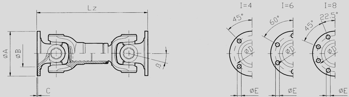
Kurzausführung mit Übergangsflansch Short design, large flange diameter
