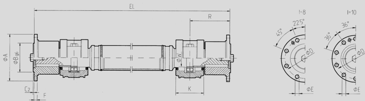
Gelenkwellenmittelteil Midship shaft
