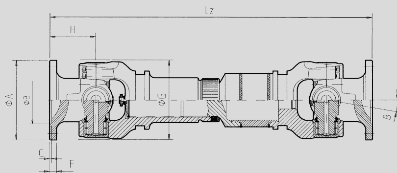
Normalausführung Standard design
