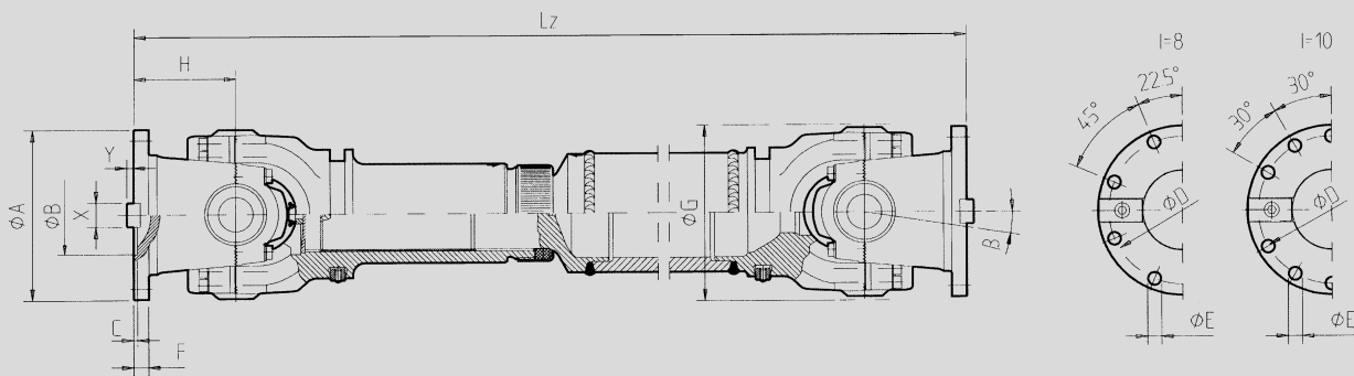
Normalausführung - Querkeilanschluss Standard design - face key connection
