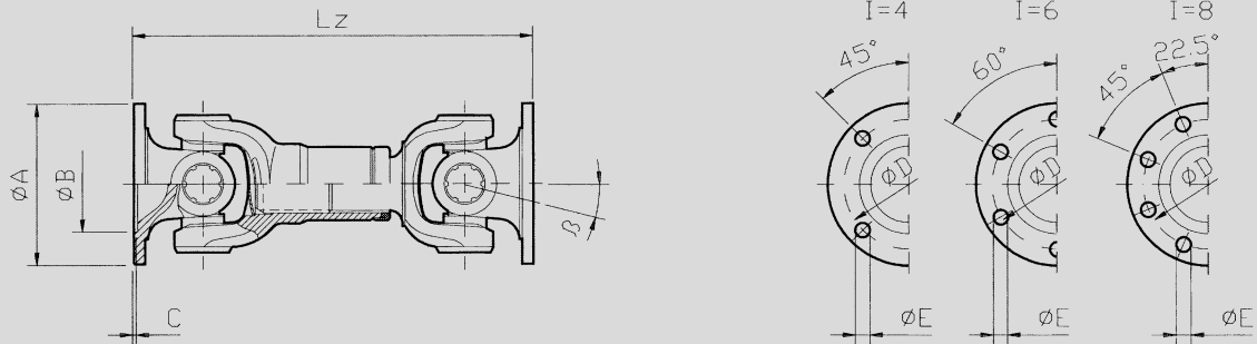
Kurzausführung Short design
