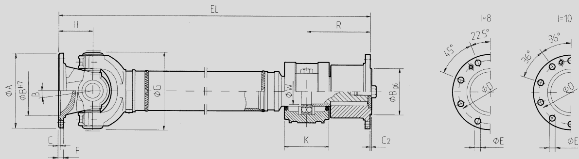
Zwischenwelle ohne Längenausgleich Intermediate shaft without length compensation
